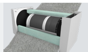
Dezentrale Wohnraumlüftung
