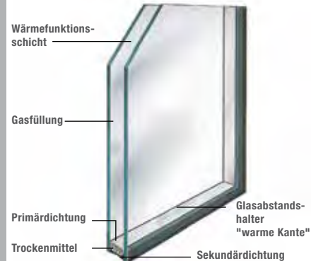
Wärmeschutzglas U g 1,1 mit 1 x Randverbund "warme Kante"
