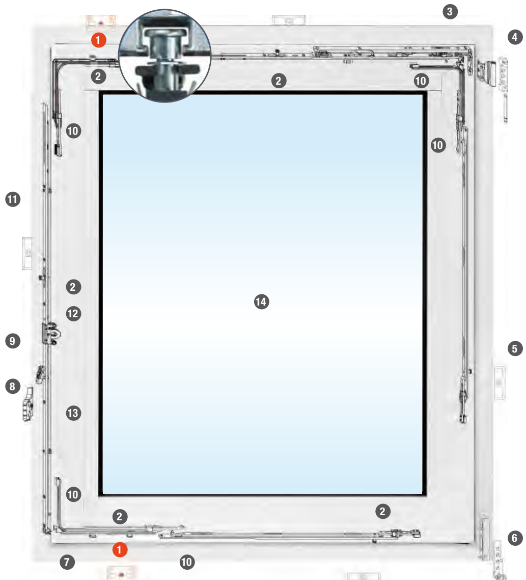
1 + 2 Pilzkopfverriegelung
